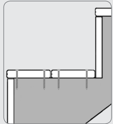
Pose basique d'un escalier
